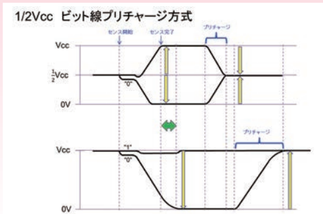
従来Vccビット線プリチャージ方式
