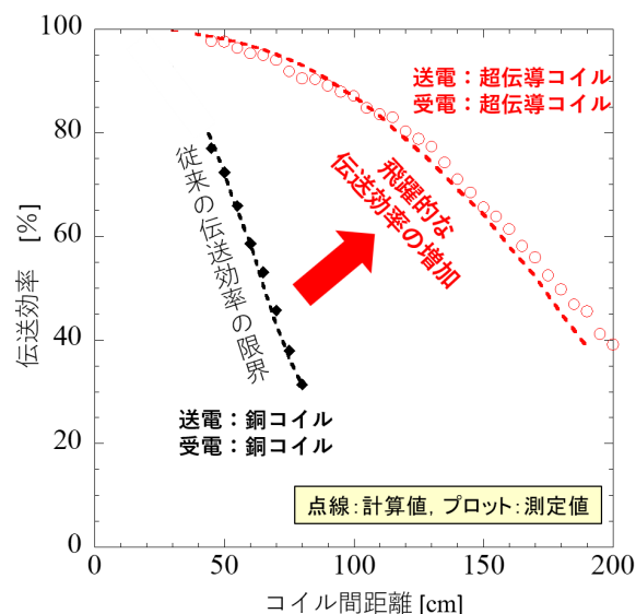
図 1 超伝導 WPT と銅 WPT の伝送効率の比較
