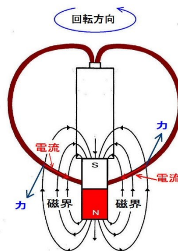
フレミングの左手の法則
